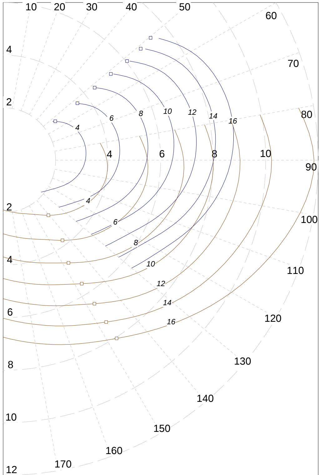
B1(L40) Polar Diagram
